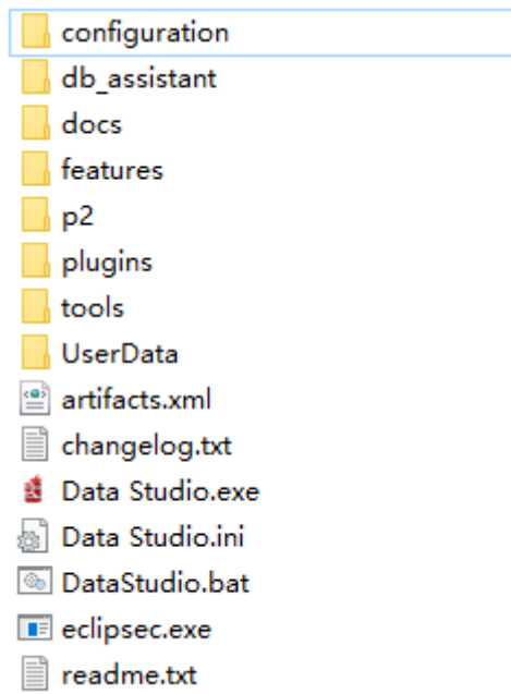
图 2-2 启动客户端
