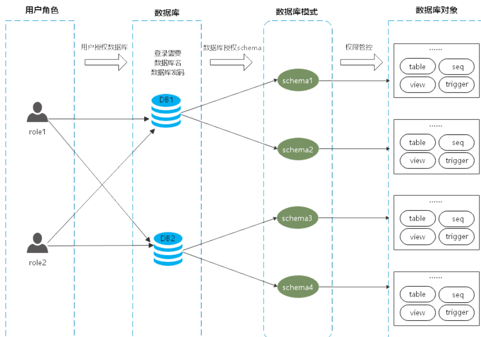
图 12-3 权限控制
