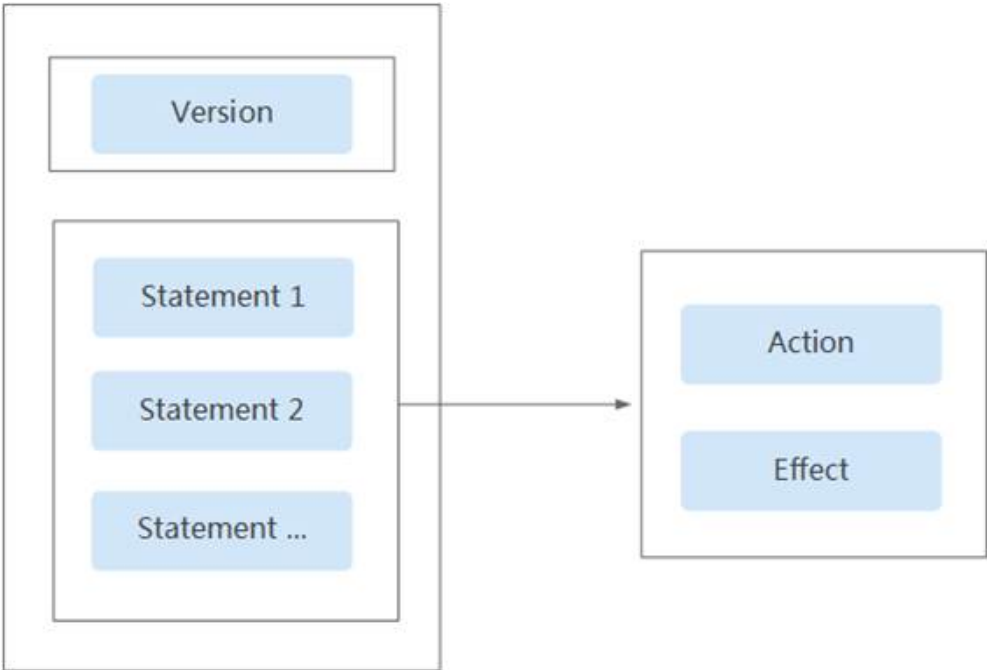
图 4-1 策略结构
